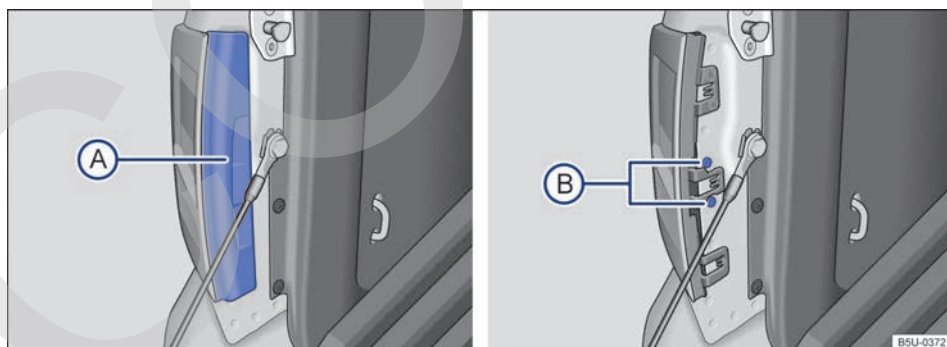
Fig. 152 En el compartimento de carga: A desinstalar la cubierta, B retirar los tornillos de fijación.
