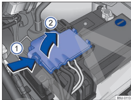
Fig. 164 Compartimento del motor: acceso al terminal positivo de la batería.
