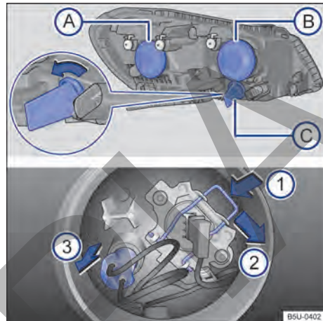
Fig. 151 En el compartimento del motor: vista trasera del faro delantero con cubierta de goma (lado izquierdo de la ilustración) - A faro bajo B faro alto y luz de posición y C indicador de dirección. Vista trasera del faro delantero sin cubierta de goma (lado derecho de la ilustración): 1 resorte de bloqueo de la lámpara incandescente del faro y 2 luz de posición.
