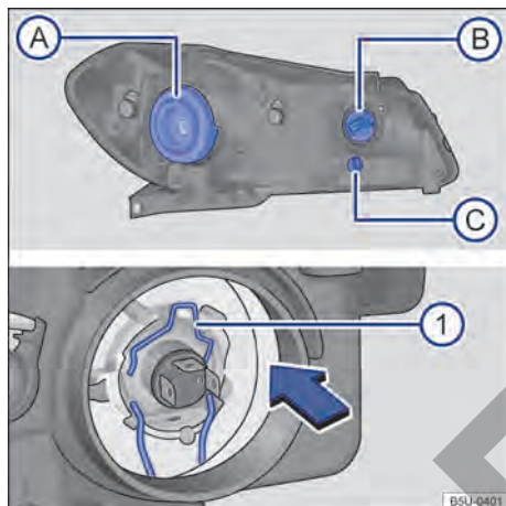
Fig. 149 En el compartimento del motor: vista trasera del farol delantero con cubierta de goma (lado izquierdo de la ilustración): A farol bajo / alto B indicadores de dirección y C luz de posición. Vista trasera del farol delantero sin cubierta de goma (lado derecho de la ilustración): 1 resorte de bloqueo de la lámpara incandescente del farol bajo/farol alto.
