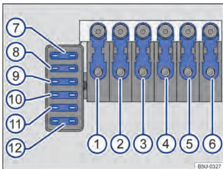
Fig. 161 Caja de fusibles.
