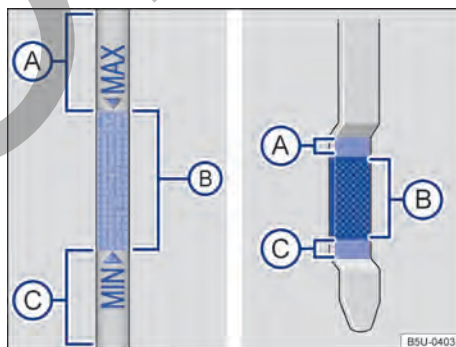
Fig. 169 Varilla de medición del aceite con marca de nivel de aceite del motor. ▶
