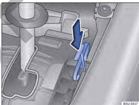
Fig. 84 Desinstalar la cubierta de la palanca selectora y desbloquear el bloqueo de la palanca selectora de emergencia.
