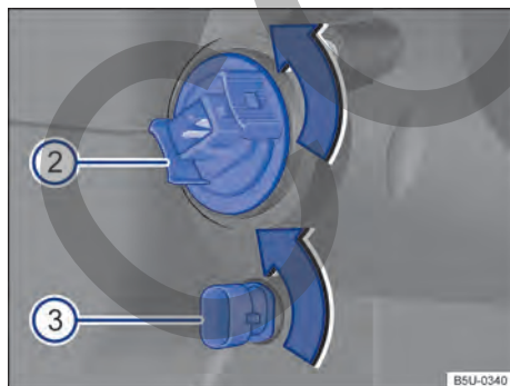
Fig. 150 En el compartimento del motor: vista trasera del farol delantero 2 indicadores de dirección y 3 luz de posición.
