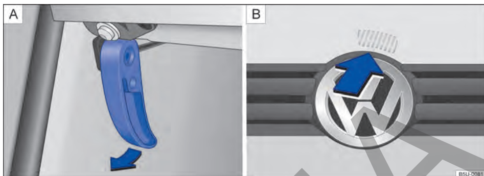
Fig. 166 [A] Palanca de desbloqueo de la tapa del compartimento del motor en la zona reposapiés del conductor. [B] Palanca de desbloqueo en la parte interior de la tapa del compartimento del motor.
