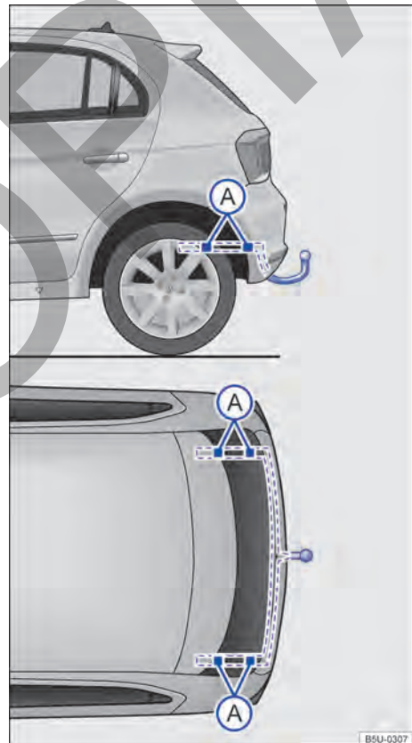
Fig. 142 Puntos de fijación para el montaje posterior de un enganche para remolque. ▶
