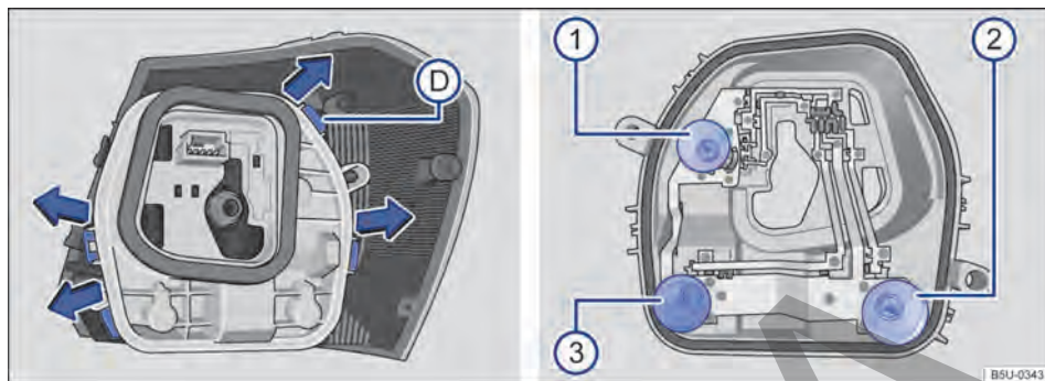
Fig. 155 Luz trasera: D desmontar el portalámparas y 1, 2 y 3 desmontar las bombillas.
