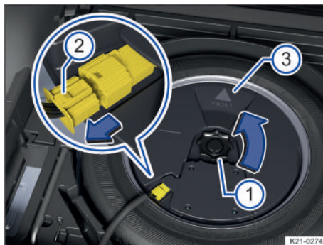
Fig. 189 En el maletero: desmontar el subwoofer (variante 2).
