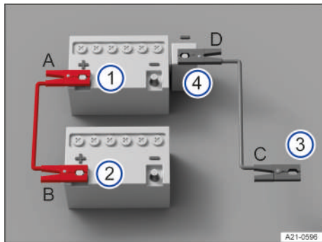
Fig. 164 Esquema para la conexión de los cables de arranque.
