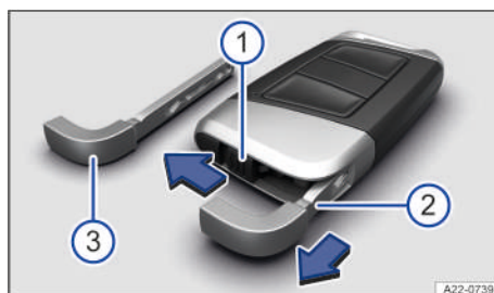
Fig. 44 Llave del vehículo: desbloqueo de la llave de emergencia (representación esquemática).
