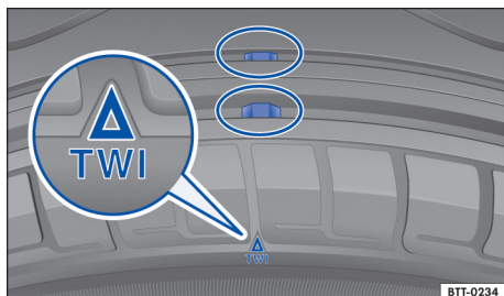
Fig. 192 Perfil del neumático: indicadores de desgaste.
