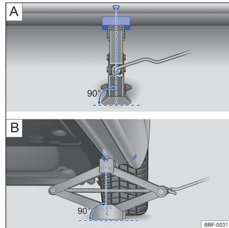
Fig. 197 Puntos de apoyo del gato y gato posicionado atrás en el lado izquierdo trasero del vehículo.
