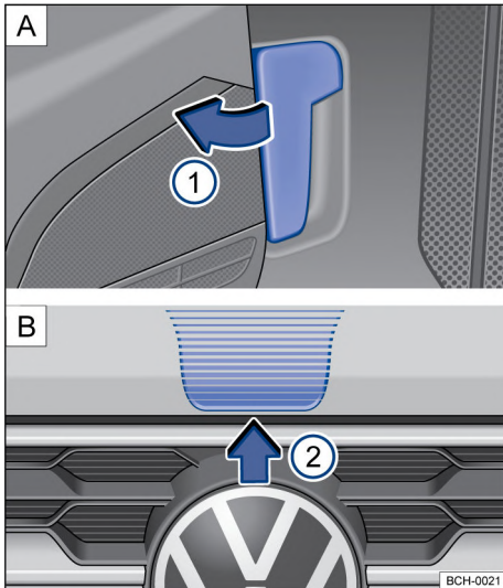
Fig. 178 [A] Palanca de desbloqueo de la tapa del compartimento del motor en la zona reposapiés del conductor. [B] Palanca de desbloqueo en la parte interior de la tapa del compartimento del motor.
