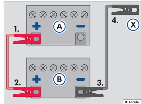
Fig. 177 Esquema para la conexión de los cables auxiliares de arranque de batería del vehículo descargada (A) y batería del vehículo que provee la corriente (B).
