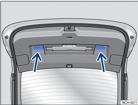
Fig. 59 Tapa trasera abierta: cavidades (flechas) para tirar y cerrar.
