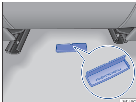
Fig. 202 Delante del asiento del pasajero trasero en el piso derecho: número de identificación del vehículo (número de bastidor).
