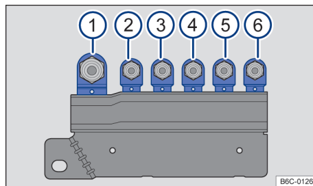
Fig. 173 En el compartimento del motor encima de la batería: disposición de los fusibles.
