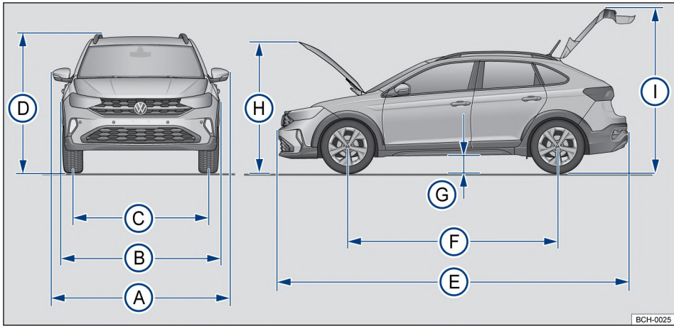
Fig. 205 Dimensiones.
