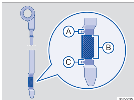
Fig. 182 Varilla de medición del aceite con marca de nivel de aceite del motor.
