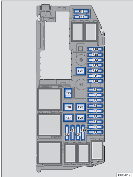
Fig. 172 En el compartimento del motor: disposición de los fusibles.
