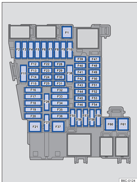
Fig. 170 En el panel de instrumentos: disposición de los fusibles.
