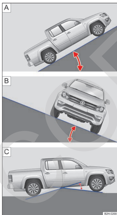
Fig. 141 Representación del ángulo de pendiente A , del ángulo de inclinación B y del ángulo ventral C .
