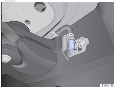
Fig. 137 En los bajos del vehículo, en el larguero: tornillo de desagüe.
