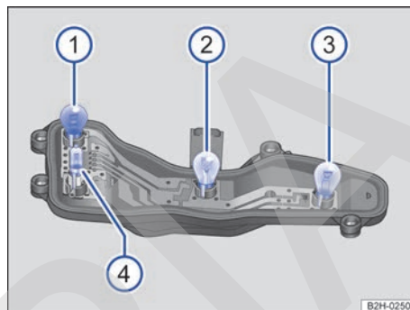
Fig. 200 Portalámparas.
