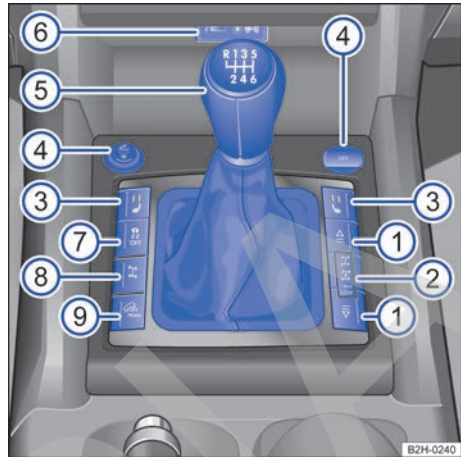
Fig. 10 Cuadro general de la parte delantera de la consola central (vehículos con el volante a la derecha).
