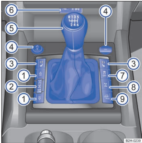
Fig. 9 Cuadro general de la parte delantera de la consola central (vehículos con el volante a la izquierda).
