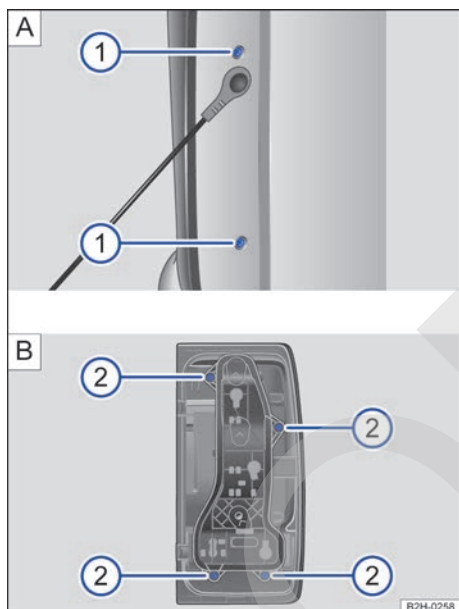
Fig. 200 Portalámparas.
