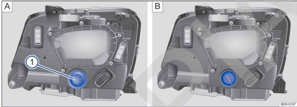
Fig. 196 En el compartimento del motor: tapa del faro derecho de xenón: 1 Luz de giro
