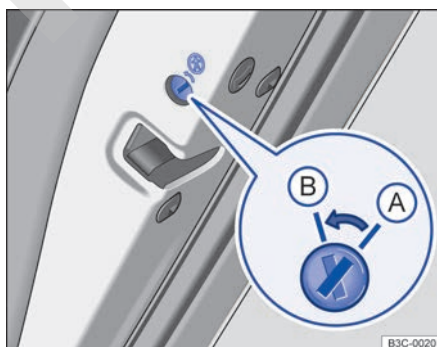
Fig. 23 En la puerta trasera derecha: seguro para niños (A) desactivado, (B) activado.
