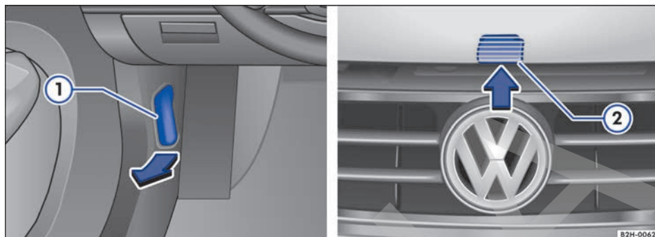
Fig. 147 ⓘ En la zona reposapiés del conductor: palanca de desbloqueo del capó del motor. ⓘ Palanca de desbloqueo para apertura del capó del motor, en la parrilla del radiador.
