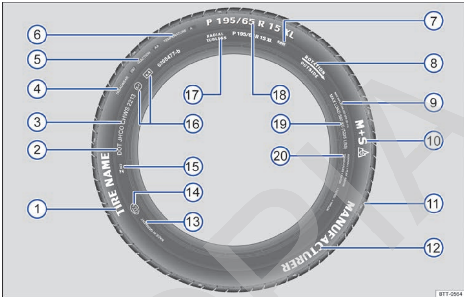
Fig. 162 Inscripciones internacionales en los neumáticos.
