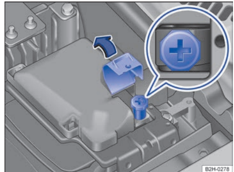
Fig. 207 En el lado izquierdo del compartimento del motor: toma para la ayuda de arranque (polo positivo).
