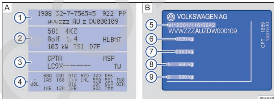
Fig. 213 A) Etiqueta portadatos del vehículo: en la figura, por ejemplo, con letras distintivas del motor CPTA B) Placa de modelo.
