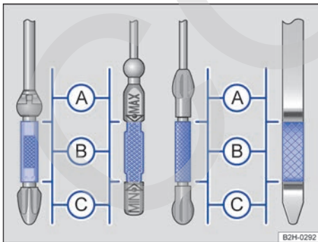
Fig. 149 Varilla de medición con marcas del nivel de aceite del motor.
