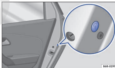
Fig. 168 En el frontal de la puerta trasera derecha: bloqueo de emergencia tapado por una junta de goma.
