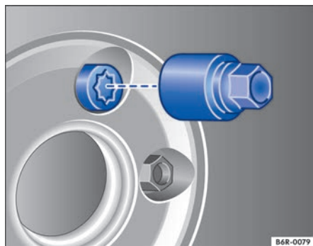
Fig. 182 Cambio de rueda: tornillo de rueda antirrobo y adaptador.
