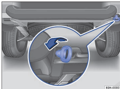
Fig. 212 En el lado derecho del paragolpes trasero: gancho para remolque enroscado.
