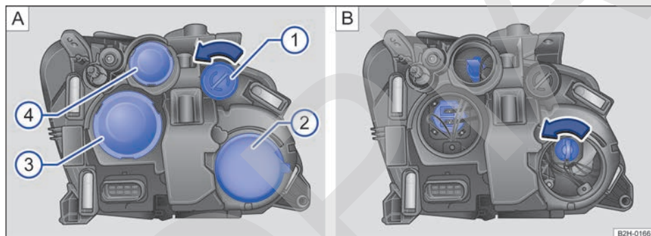
Fig. 195 En el compartimento del motor: tapas del faro izquierdo. ① Luz de giro, ② luz alta y luz diurna, ③ luz baja, ④ luz de posición.
