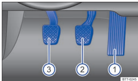
Fig. 110 Pedales en los vehículos con cambio manual: ① acelerador, ② freno, ③ embrague.
