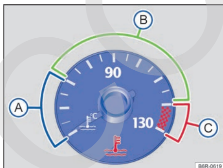
Fig. 151 Indicador de la temperatura del líquido refrigerante del motor en el tablero de instrumentos: (A) zona fría; (B) zona normal; (C) zona de advertencia.
