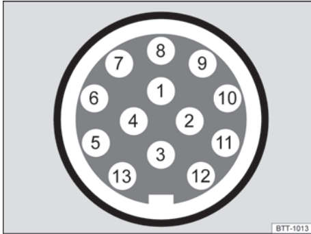
Fig. 94 Representación esquemática: asignación de los pines de la toma de corriente para remolque.
