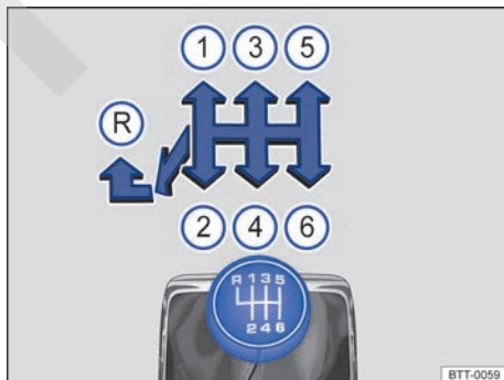
Fig. 112 Esquema de las marchas de un cambio manual de 6 marchas.
