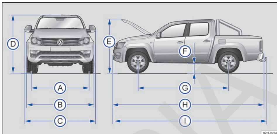
Fig. 215 Dimensiones.
