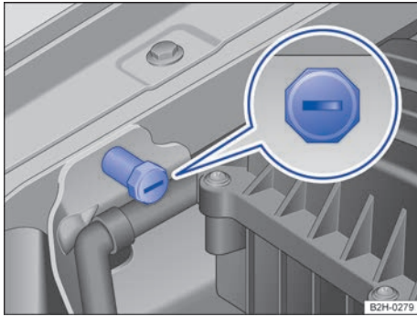
Fig. 208 En el lado derecho del compartimento del motor: toma para la ayuda de arranque (polo negativo).
