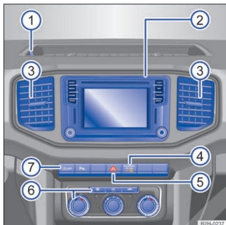
Fig. 8 Cuadro general de la parte superior de la consola central (vehículos con el volante a la izquierda).
