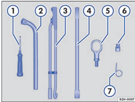
Fig. 174 Piezas de las herramientas de a bordo.
